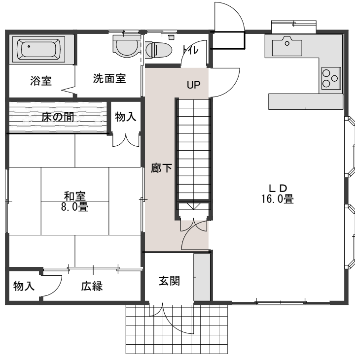
1階 縮尺 1/100
